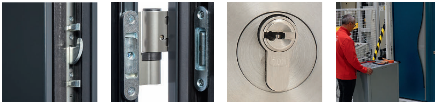
Détail des renforts sur une porte Aluminium
